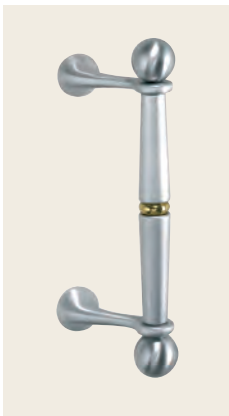
HA 5010 Stoßgriff 300 mm Chrom matt, Kombination mit Zierring, Messing poliert
