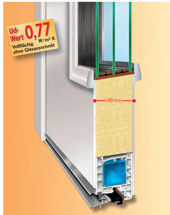
EcoDoor 8.0 Plano mit innerem und äußerem Vollblatt-Design Kunststoff-Haustüren in zeitloser, eleganter Optik Bautiefe 88 mm
