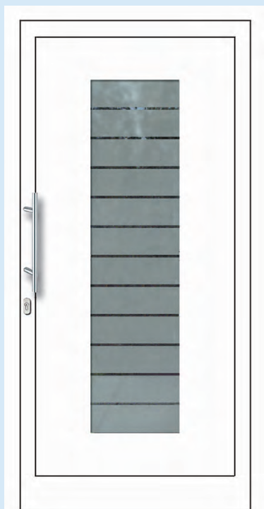
Kunststoff Modell 20299 (PG30) Aluminium Modell 40299 (PG32) Variante: Classic Glas: „Arnheim“, Klarglas mit Teilmattierung Griff: HA1039-40 Edelstahl PZ-Rosette: HA1075 Edelstahl (oval)
